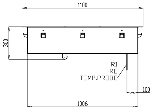
Front aanzicht
